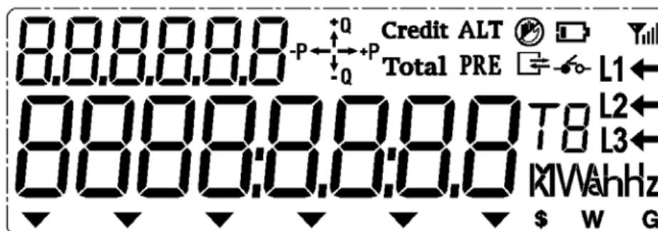
Рисунок 16. Общий вид ЖКИ счетчика АИСТ А100-Н
