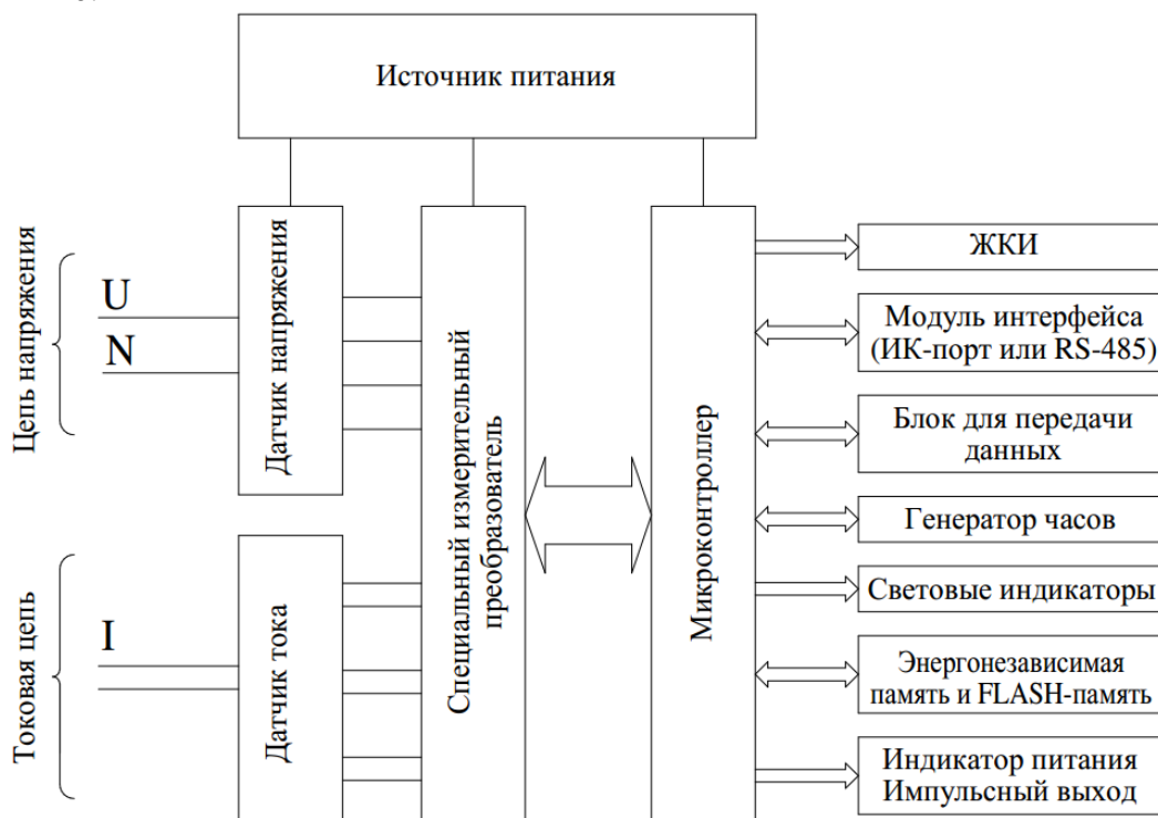
Рисунок 10. Структурная схема счетчика
