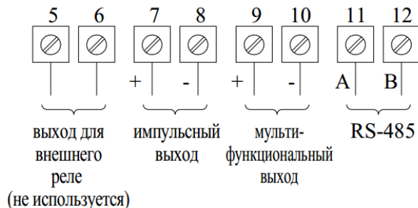
Рисунок 6. Клеммная колодка счетчика АИСТ А100-Н
