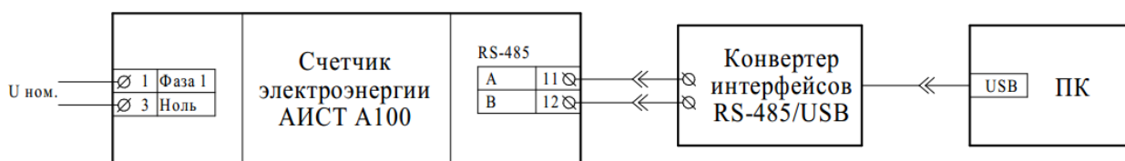
Рисунок 11. Схема подключения счетчиков к компьютеру
