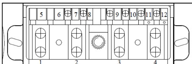
Рисунок 6. Клеммная колодка счетчика АИСТ А100-Н
