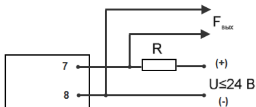
Рисунок 9. Подключение к испытательному выходному устройству
