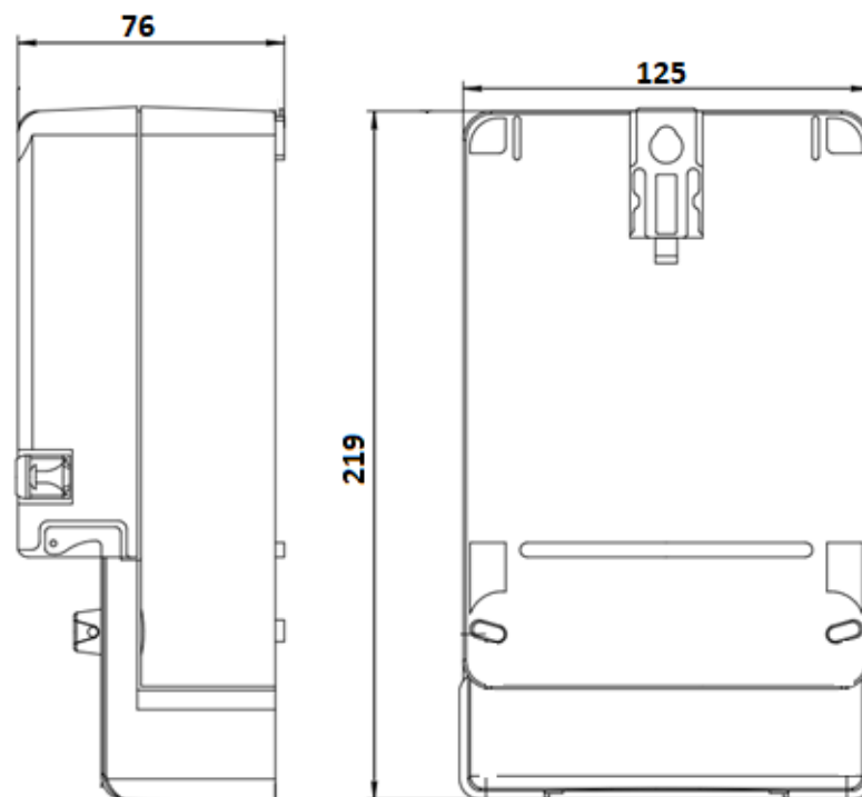
Рисунок 3. Габаритные размеры АИСТ А100-Н
