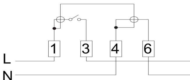
Рисунок 8. Вид клеммной колодки и схема подключения счетчика АИСТ А100- Н
