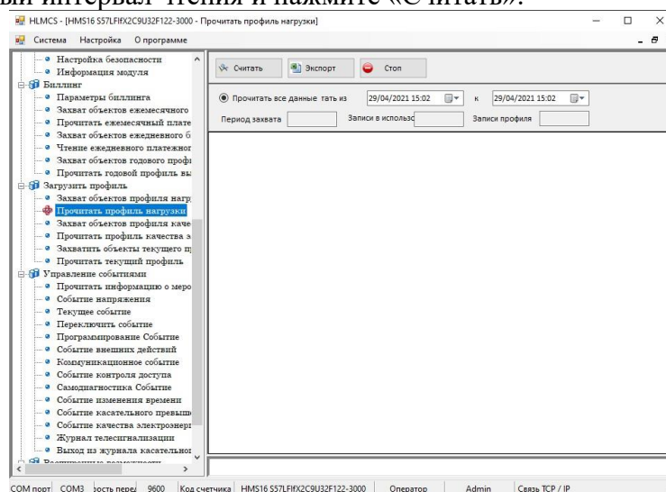
Рисунок 14. Раздел «Профиль мощности» конфигуратора счетчика АИСТ А100-Н
